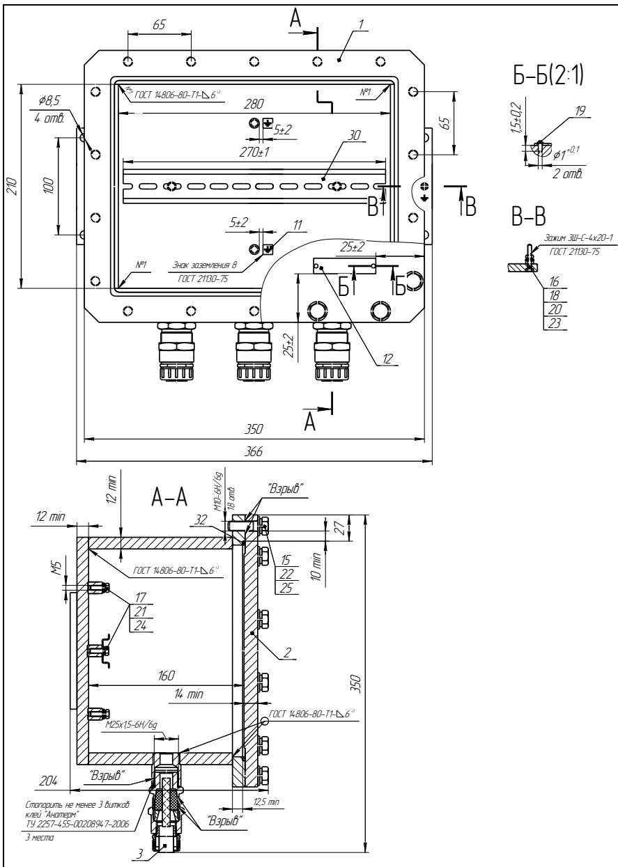
Рисунок. Б.1 – Чертеж средств взрывозащиты КС
